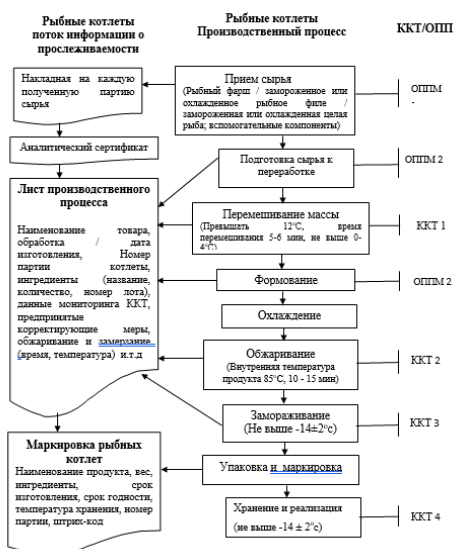
Рисунок 8. Процесс разработки рыбных котлет и поток информации о прослеживаемости, критическая контрольная точка - ККТ, Оперативная предупредительная программа - ОППМ
