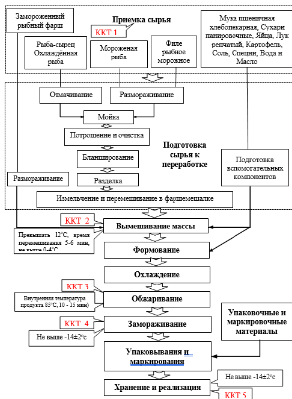
Рисунок 5. Схема технологического процесса изготовления рыбных котлет.
