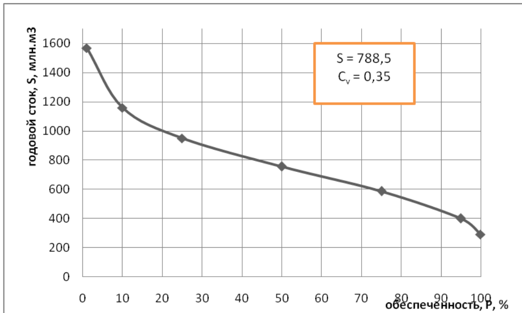
Рисунок 1 - Аналитическая кривая обеспеченности годового стока в расчетном створе
