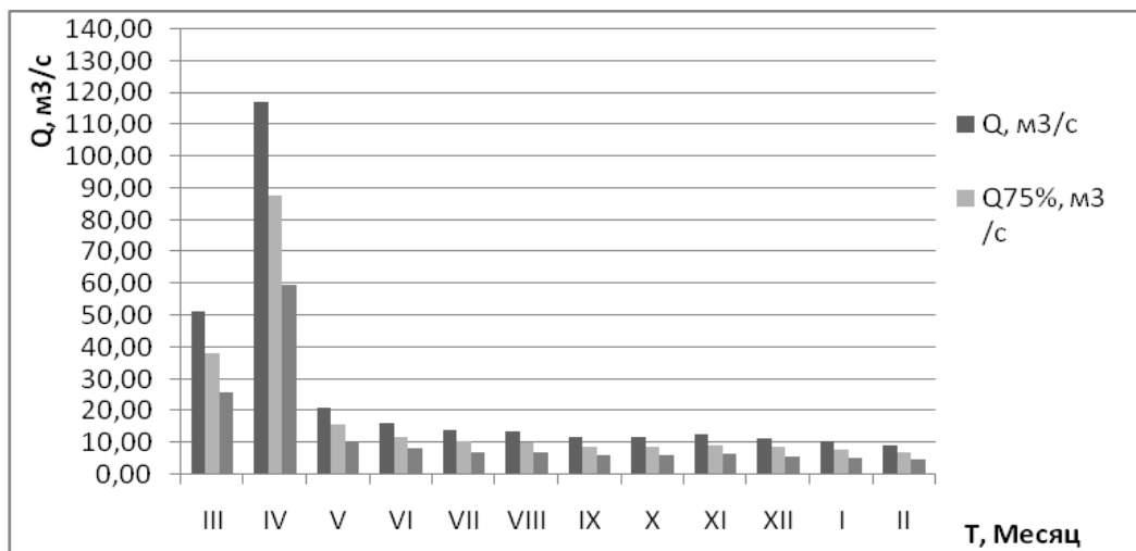
Рисунок 3 - Гидрографы среднемесячных расходов естественного стока в годы разной водности
