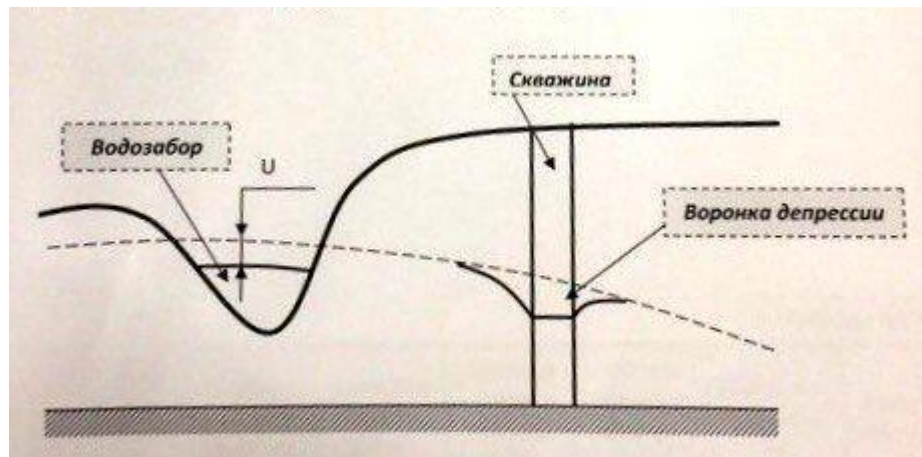
Рисунок 4 - Схема изменения ресурсов поверхностного стока при подземном водозаборе
