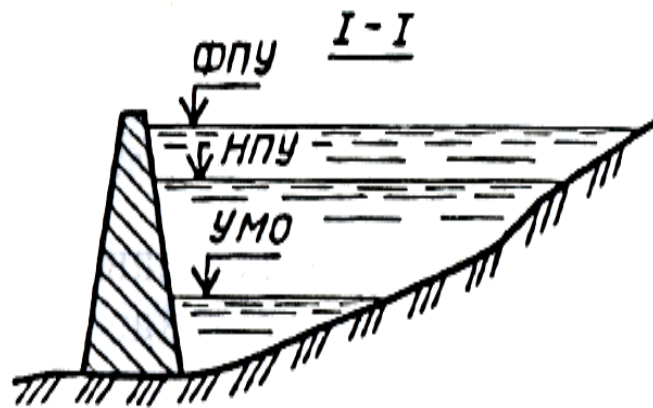
Рис.6- Уровни воды в водохранилище
