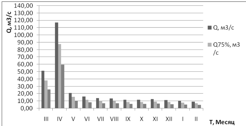
Рисунок 3 - Гидрографы среднемесячных расходов естественного стока в годы разной водности
