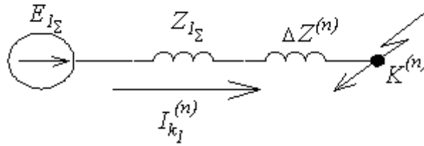
Рис.2 Схема замещения для определения любого вида несимметричного КЗ
