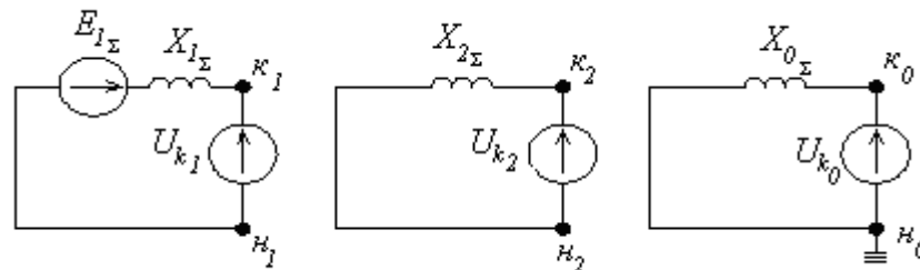
Рис.3 Схемы замещения ПП, ОП, НП
