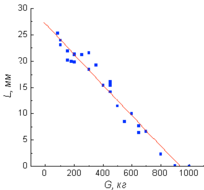
Рисунок 2.2 – Зависимость веса груза от линейных размеров
