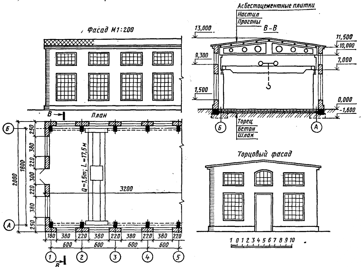
Рисунок 5.3 – Одноэтажное промышленное здание
