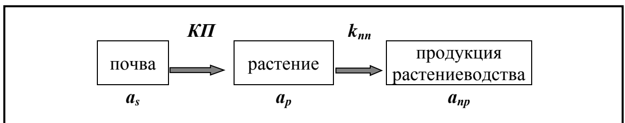
Рисунок 1 – Схема миграции радионуклида в продукцию растениеводства
