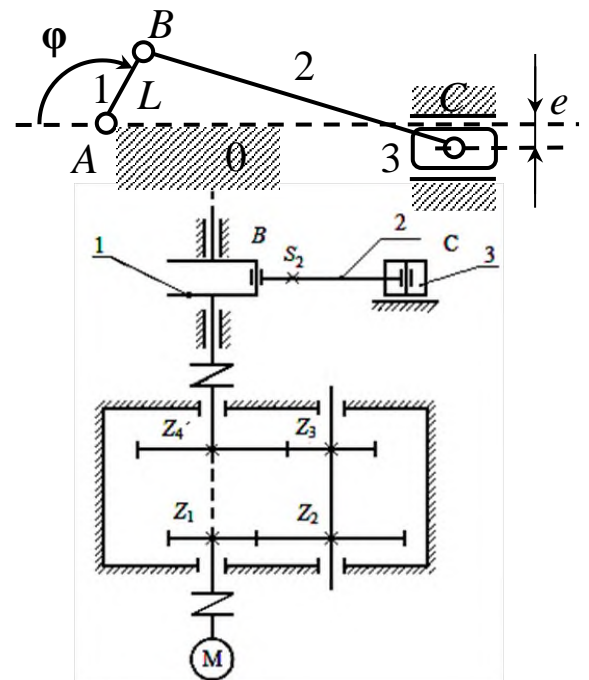
Структурные схемы привода и исполнительного механизма
