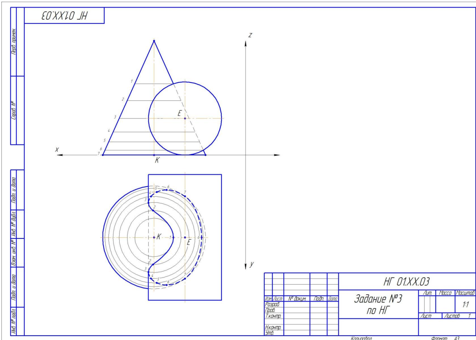
Рис. 5. Образец выполнения расчетно-графической по разделу «Начертательная геометрия». Тема ««Главные позиционные задачи»»
