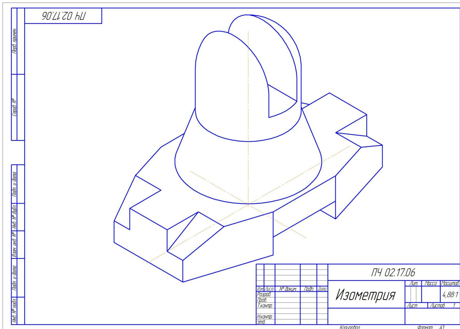
Рис. 11. Расчетно-графическая работа по разделу «Инженерная графика». Тема «Проекционное черчение» (Лист 9 – Аксонометрические проекции)
