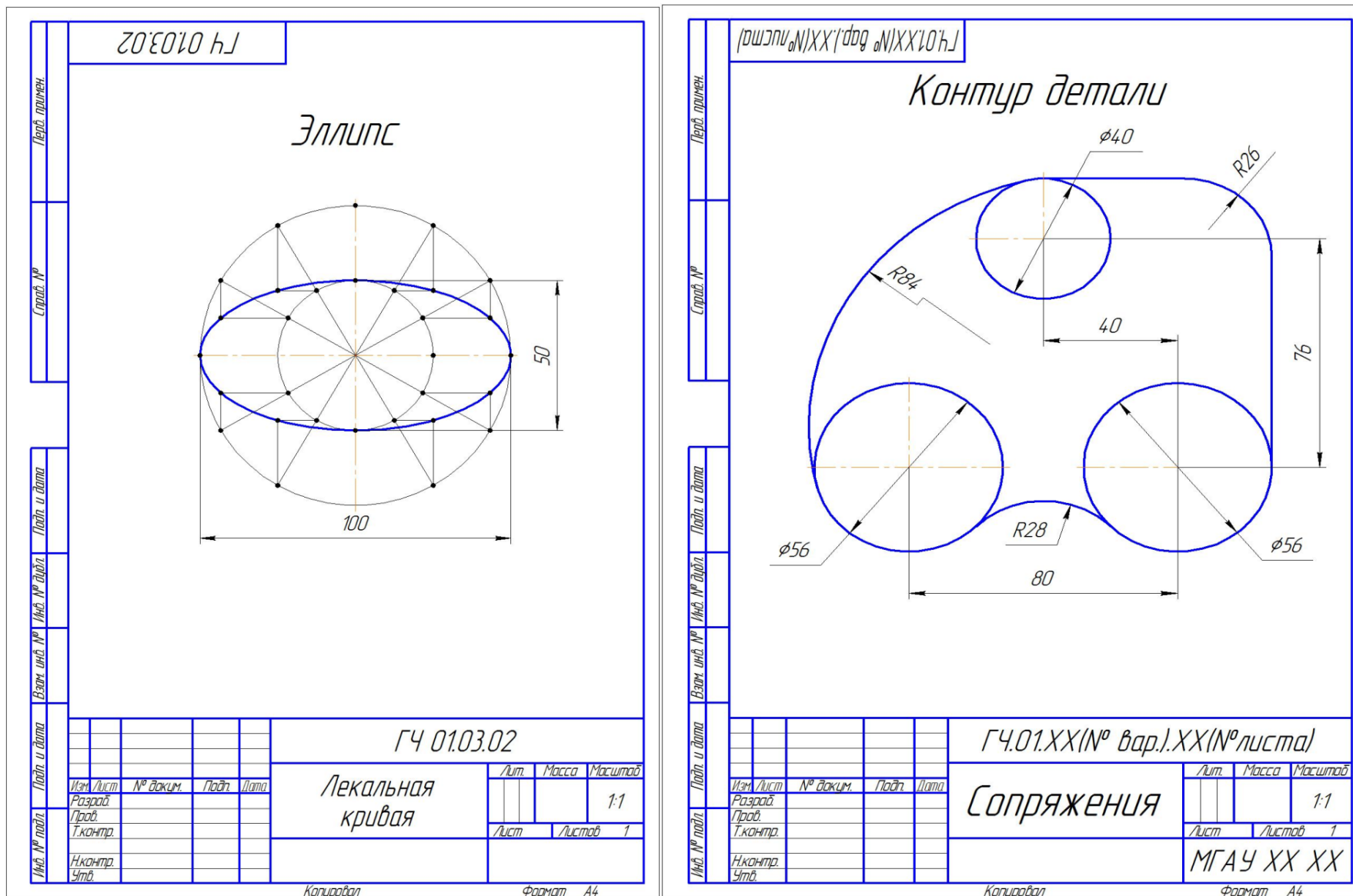
Рис. 6. Расчетно-графическая работа по разделу «Инженерная графика». Тема «Геометрическое черчение» (Лист 1 – лекальная кривая, Лист 2 – сопряжение)
