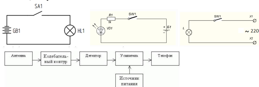
Рисунок 3.1 - Структурная схема приемника прямого усиления
