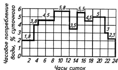
График суточного водопотребления
