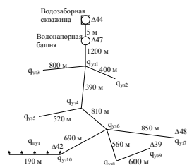
Схема систем водоснабжения
