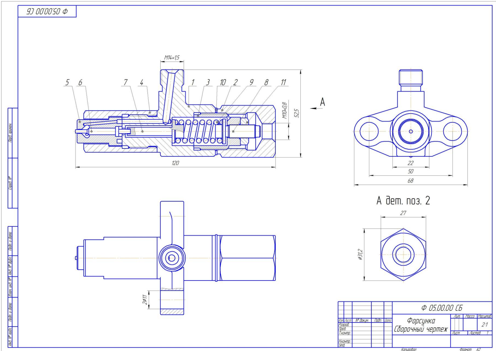
Рис. 13. Чертеж общего вида.
