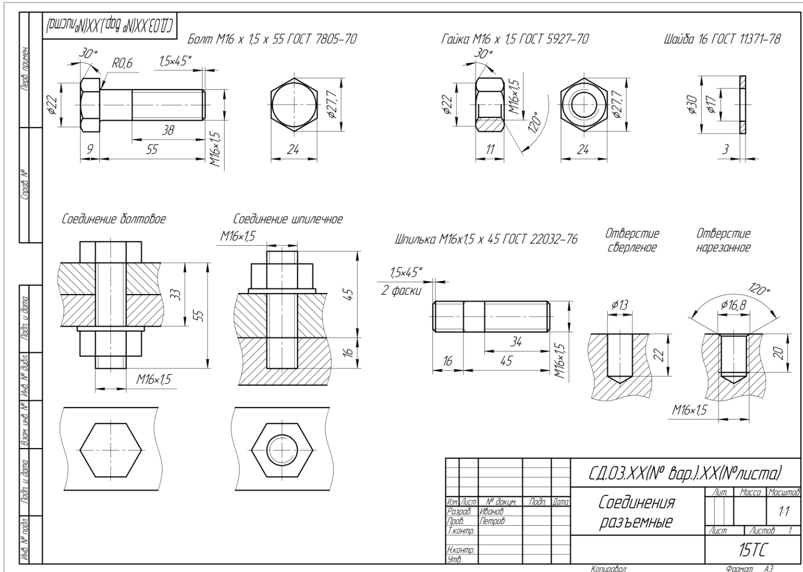
Рис. 11. Соединения разъемные резьбовые.
