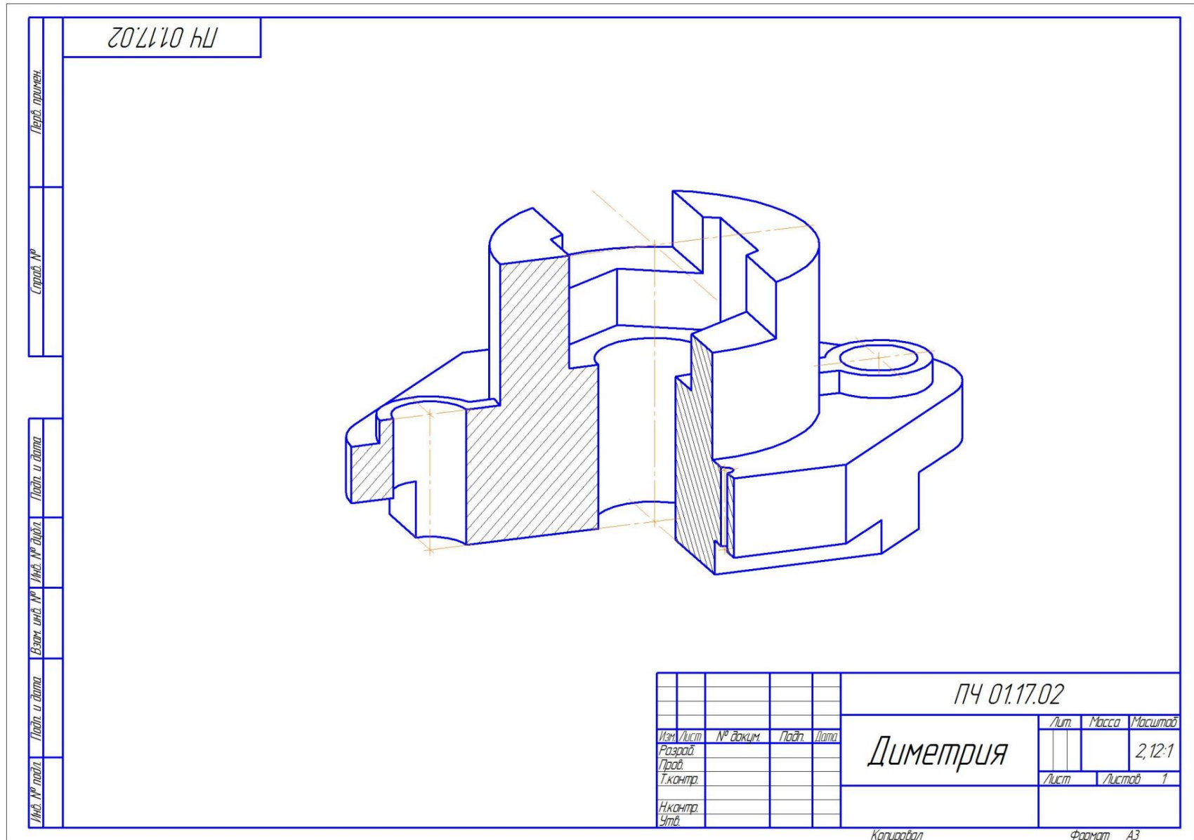
Рис.10. Прямоугольная диметрия.
