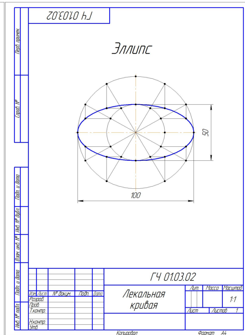
Рис. 4. Сопряжения. Лекальная кривая
