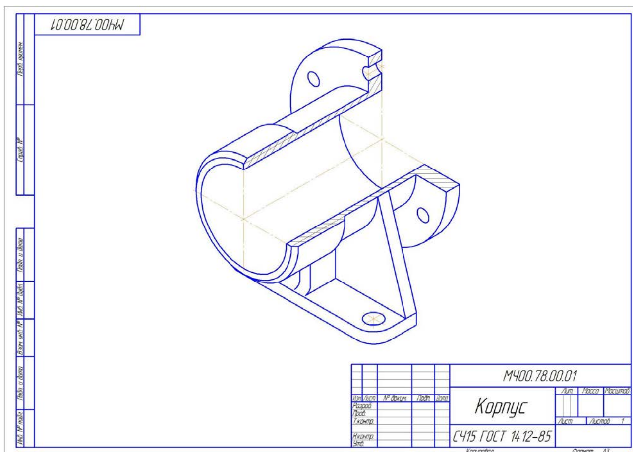
Рис. 17. Изометрия корпусной детали.
