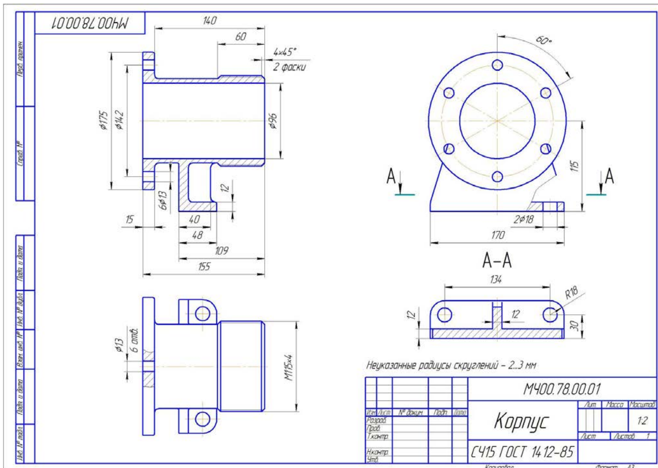
Рис. 16. «Деталирование». Чертежи деталей.
