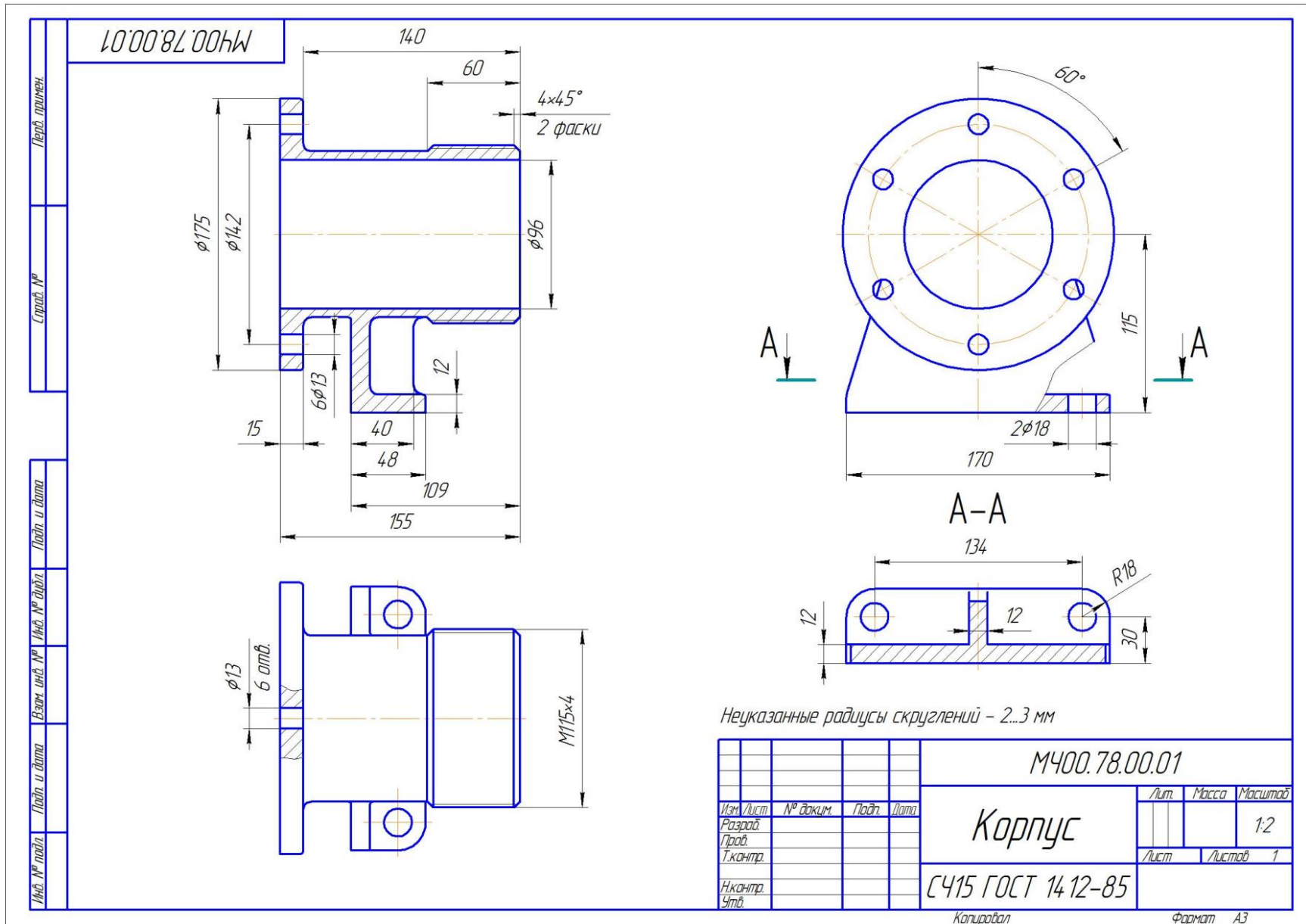
Рис. 16. «Деталирование». Чертежи деталей.
