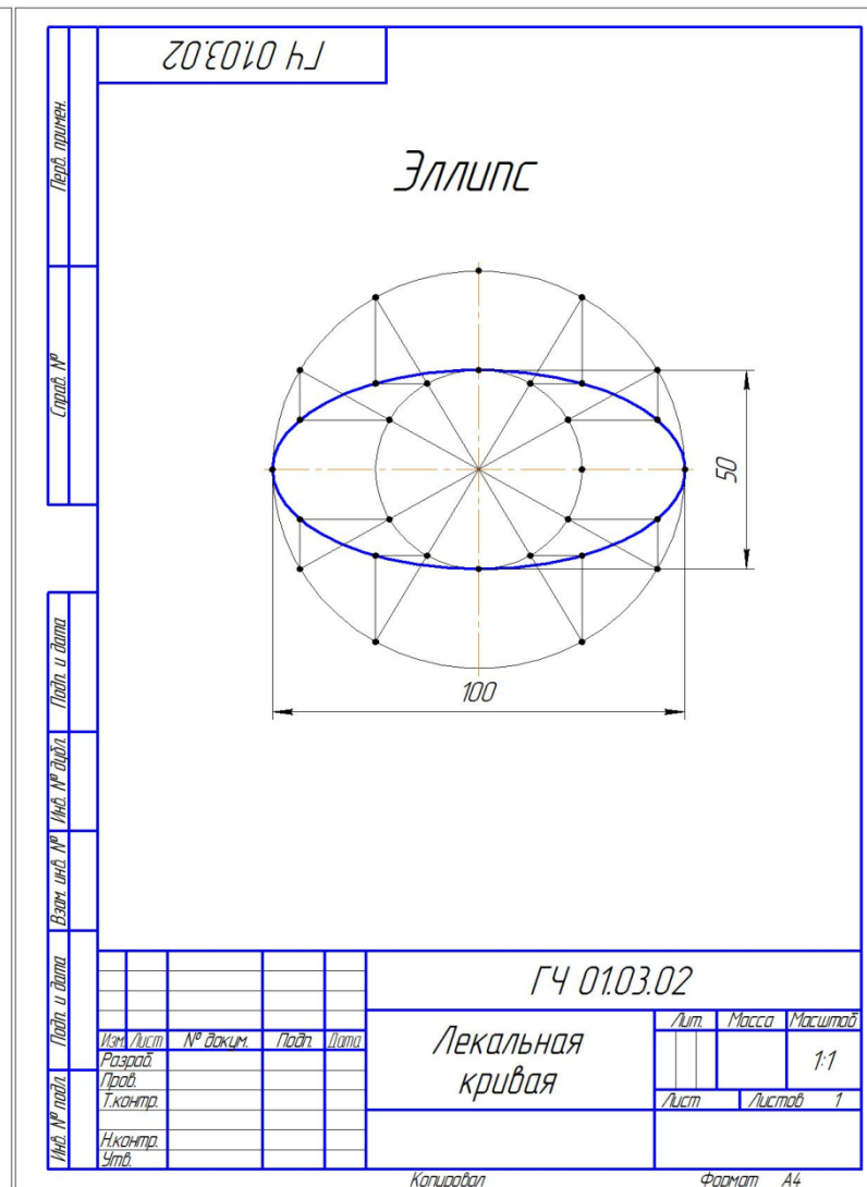
Рис. 4. Сопряжения. Лекальная кривая
