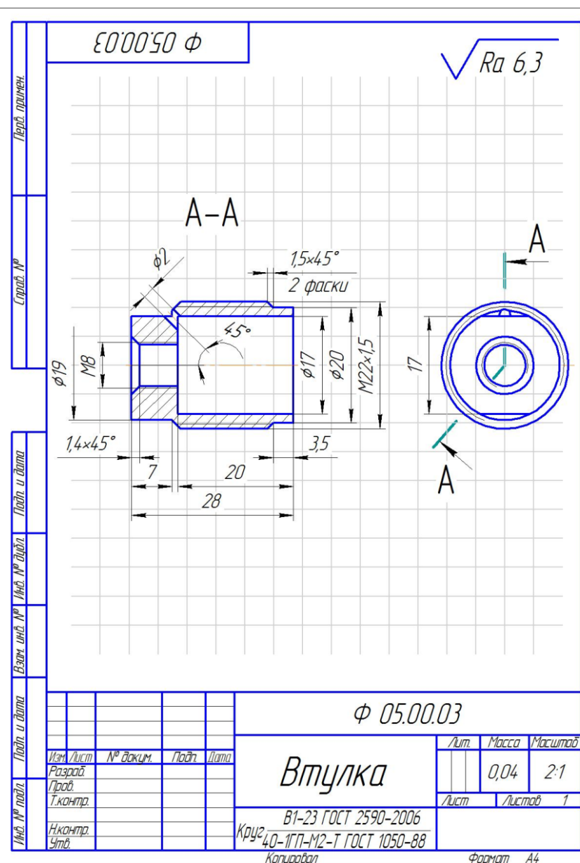
Рис. 12. Графическая работа «Чертеж общего вида» (Лист 14 – Спецификация, 15 – Эскизы деталей)
