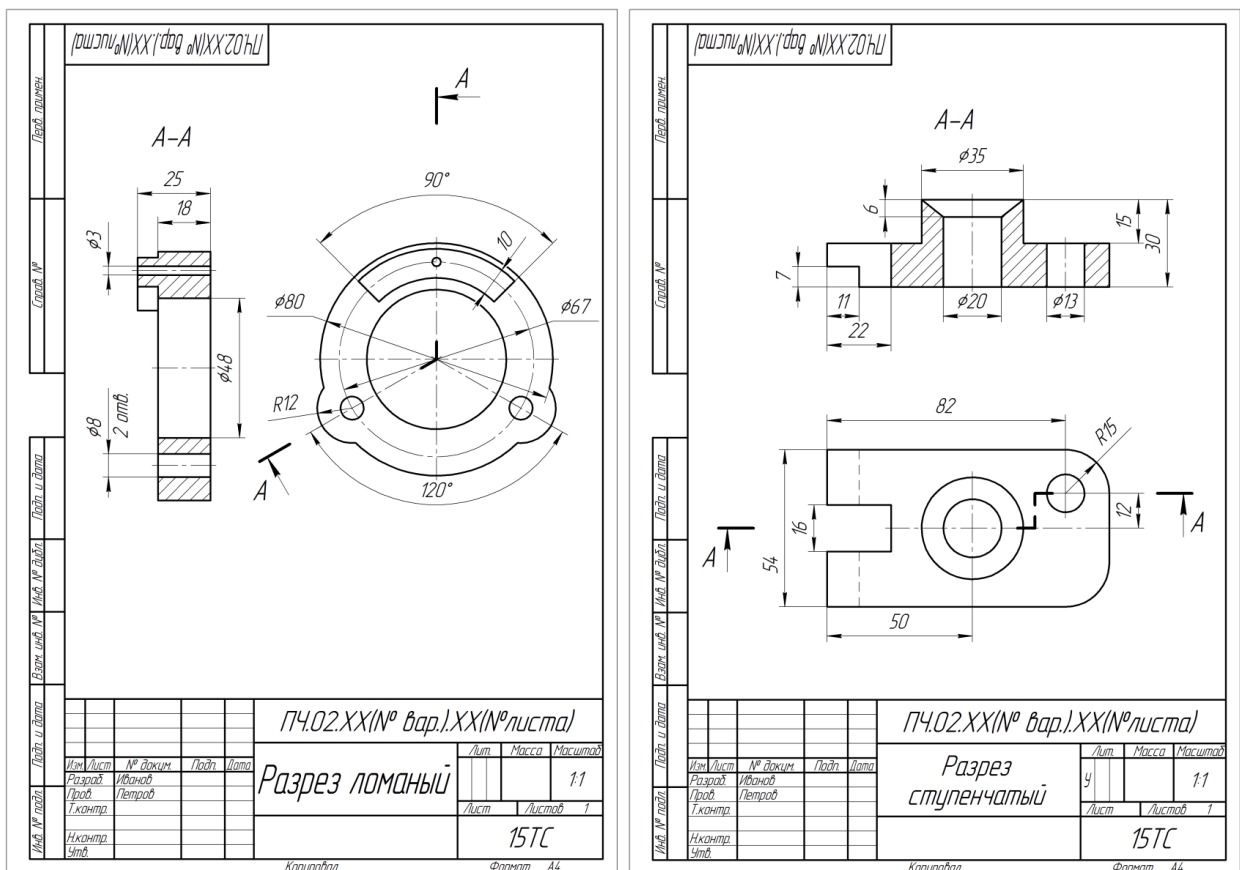
Рис. 5. Сложные разрезы.
