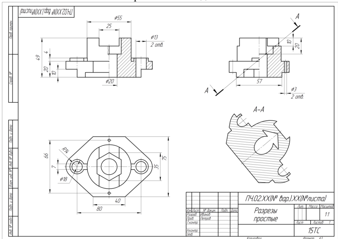
Рис. 4. Простые разрезы.
