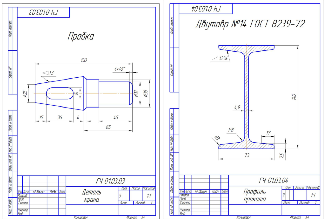
Рис. 2. Конусность. Уклон.
