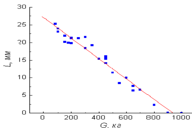
Рисунок 3.1 – Зависимость веса груза от линейных размеров
